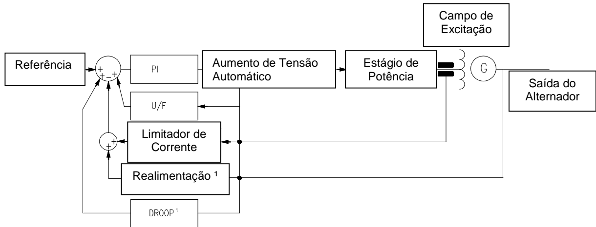
Figura 5.1: Diagrama de blocos do regulador de tensão.
