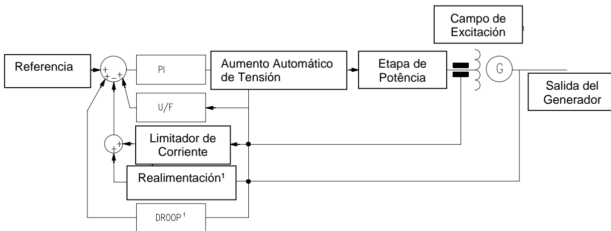
Figura 5.1: Diagrama de bloques del regulador de tensión
