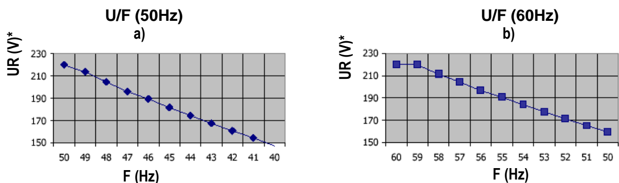
Figura 12.1: Punto de actuación de la protección U/F
