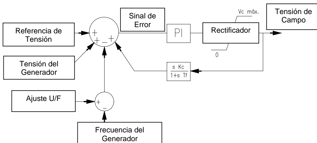
Figura 5.2: Diagrama de control del AVR-A-OPT-03
