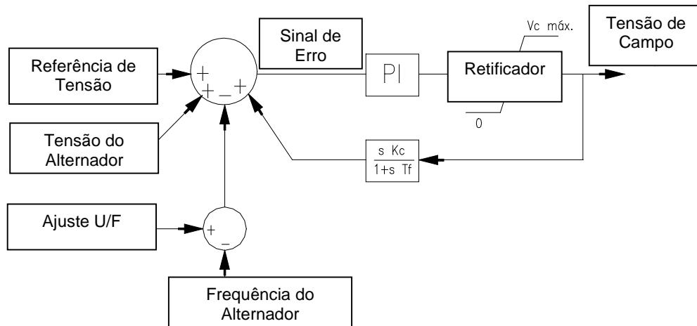
Figura 5.2: Diagrama de controle do AVR-A-OPT-03
