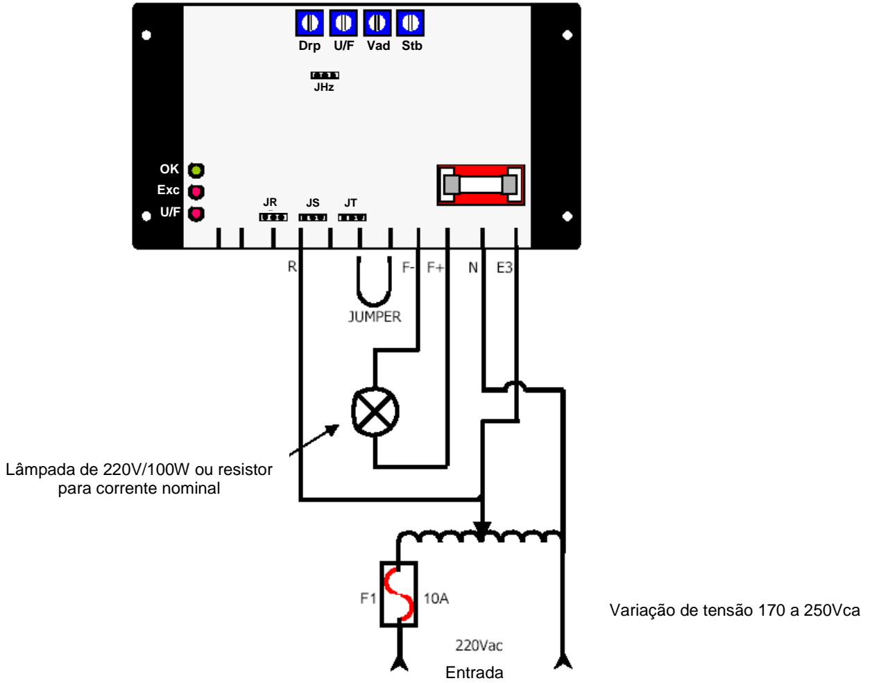
Figura 22.1: Conexão do regulador sem alternador.
