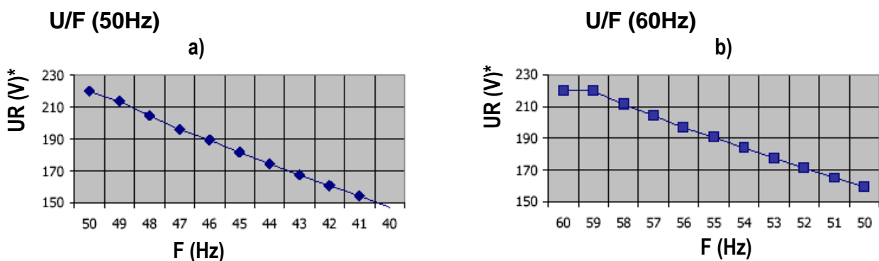
Figura 12.1: Ponto de atuação da proteção U/F.
