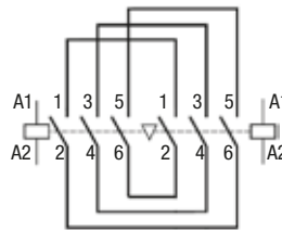
Diagrama eléctrico
