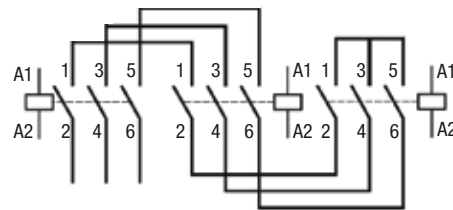
Diagrama eléctrico
